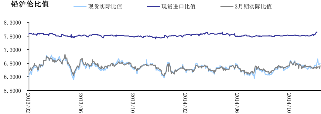
铅沪伦比值
