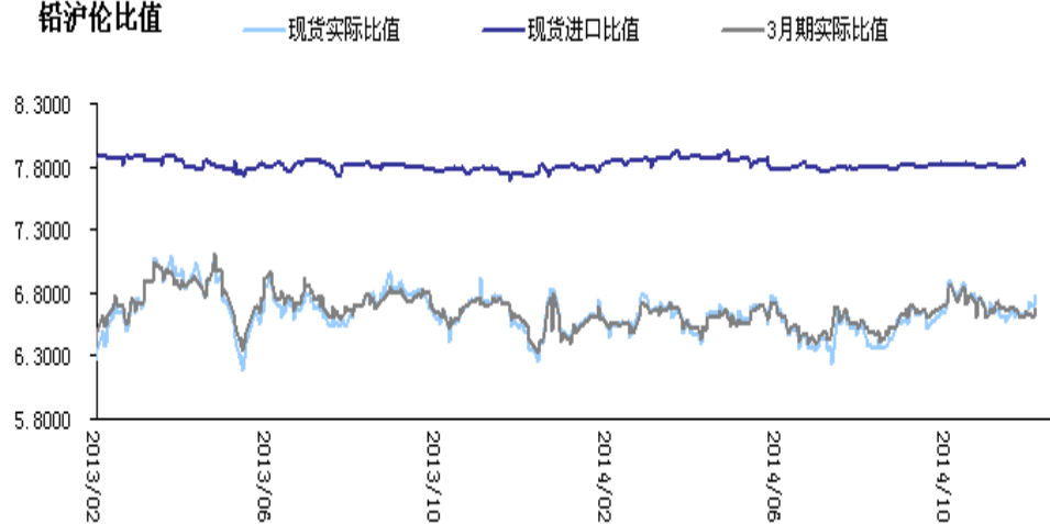
铅沪伦比值
